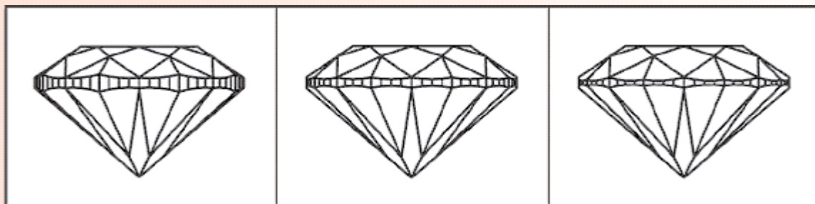
Рис. 1. Положение парных граней низа и верха относительно плоскости рундиста оказывает воздействие на форму этих граней и, следовательно, на форму рундиста.
